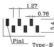
PCB Layout 线路板布局图
